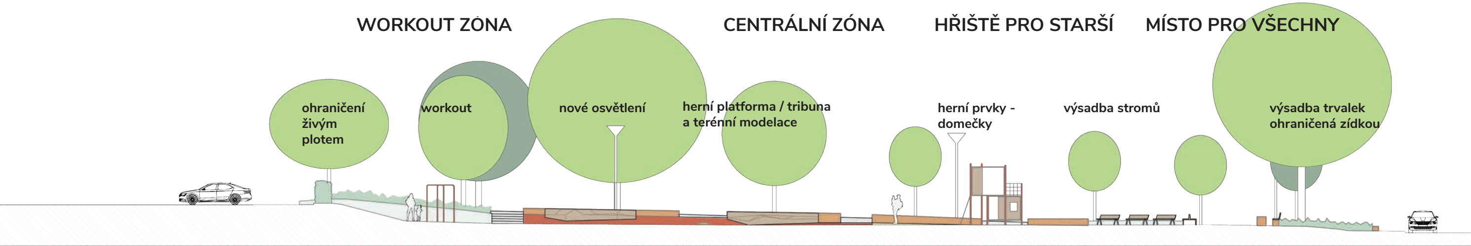
ŘEZOPOHLED BB'
